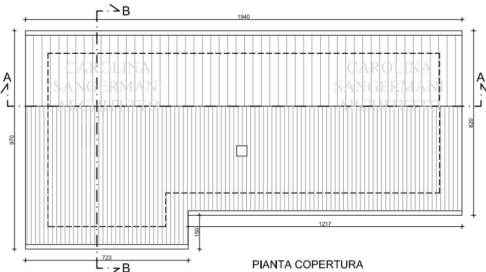
PIANTA COPERTURA
